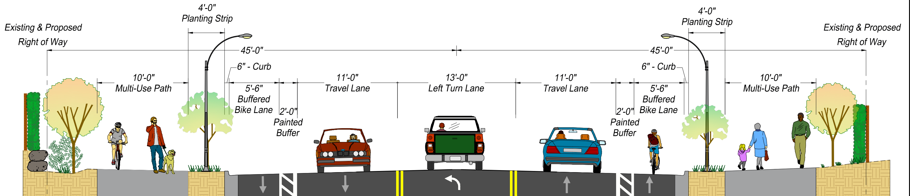
Section A-A
